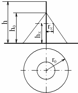
Рис. 2. Зона защиты одиночного стержневого молниеотвода
