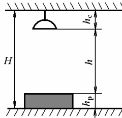
Рис. 1. Схема подвеса светильника
