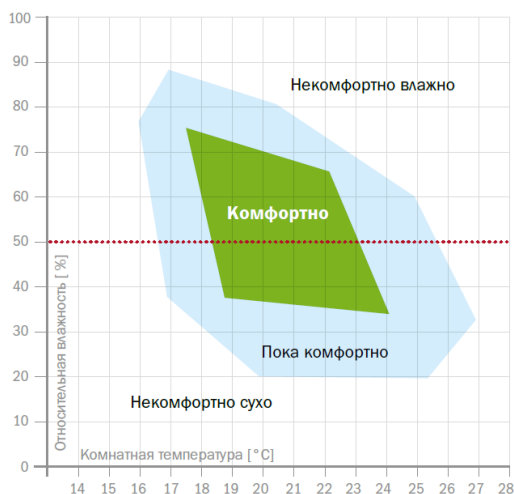
Рис. 1 Взаимосвязь комфортного пребывания в помещении от температуры и относительной влажности воздуха [6]
