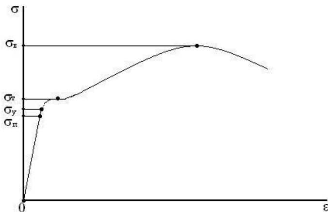
Рис. 1. Диаграмма растяжения стали
