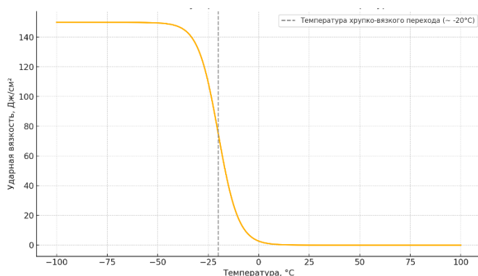
Рис. 2. Зависимость ударной вязкости стали от температуры
