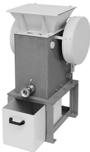
Рис. 2 – Щековая дробилка лабораторная
