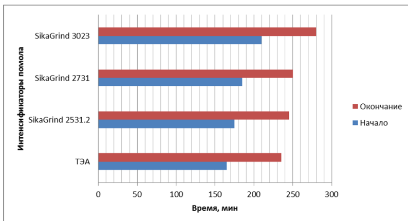
Рис. 4 - Сроки схватывания (начало и окончание) с интенсификаторами ТЭА (в дозировке 120 гр/т) и SikaGrind (в дозировке 200 гр/т)
