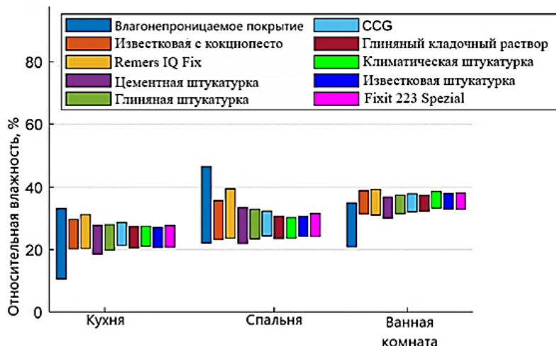
Рис. 2 – Зависимость относительной влажности воздуха от покрытия и исследуемого помещения [7]
