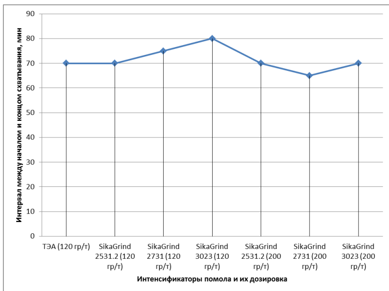
Рис. 5 – Интервал между началом и концом схватывания с различными интенсификаторами
