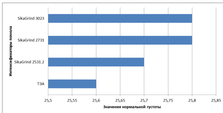
Рис. 2 - Нормальная густота с интенсификаторами ТЭА (в дозировке 120 гр/т) и SikaGrind (в дозировке 200 гр/т)
