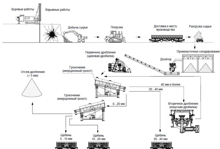
Рис. 1 – Технологическая схема получения гранитного щебня и отсева
