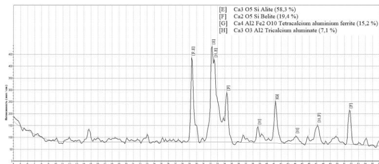
Рис. 1 Рентгенограммы исследуемых образцов: а – микроцемент «МикроОСТ»; б – портландцемент ЦЕМ I 42,5 Н
