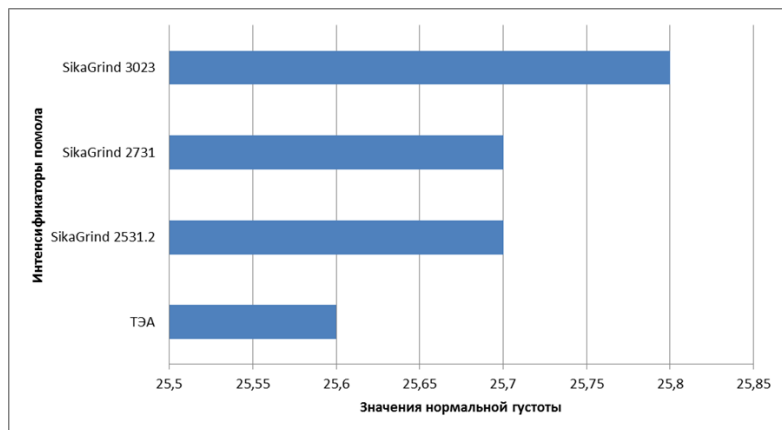
Рис. 1 - Нормальная густота с интенсификаторами ТЭА и SikaGrind (в дозировке 120 гр/т)
