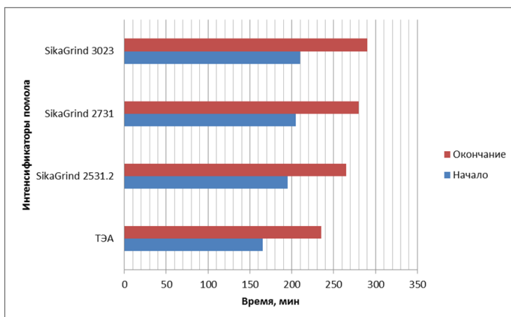
Рис. 3 - Сроки схватывания (начало и окончание) с интенсификаторами ТЭА и SikaGrind (в дозировке 120 гр/т)
